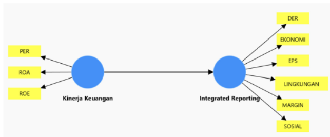
Gambar 1. Analisis Statistik PLS SEM
